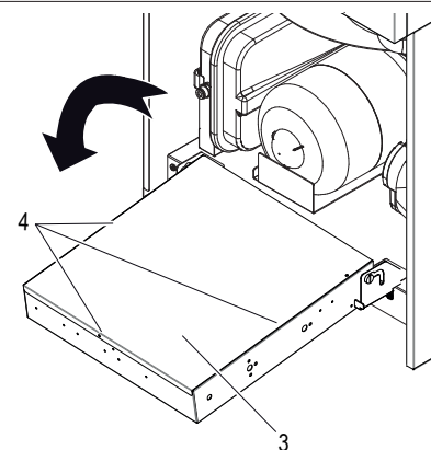
rys. 20 - jak obrócić skrzynkę elektryczną
