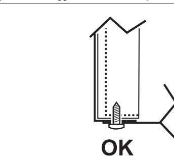
fig. 16 - montaggio con viti inferiori
