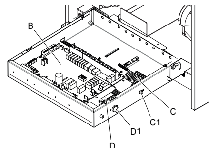
rys. 21 - widok wnętrza tablicy elektrycznej
